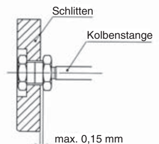
Kolbenstange und Anschluss am Tisch
