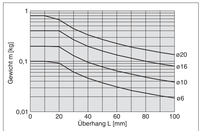
Diagramm 3 max. Geschwindigkeit 500 mm/s
